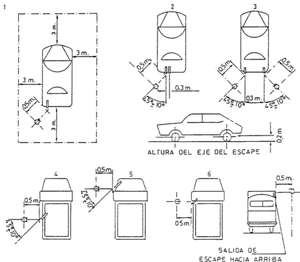
Posiciones para el ensayo de vehículos parados
