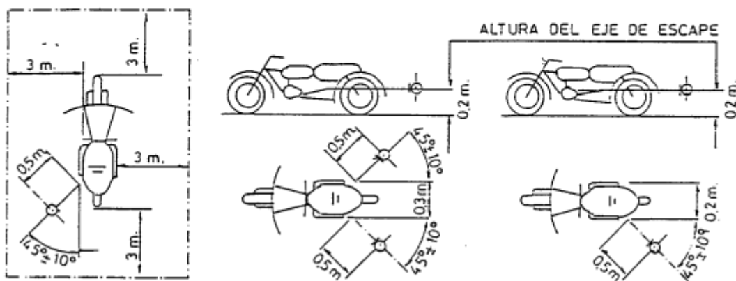
Posiciones para el ensayo de motocicletas paradas
